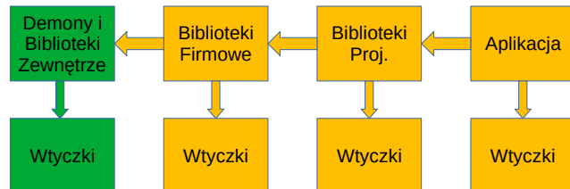
Architektura Typowego Prog. Nieuprzywilejowanego
